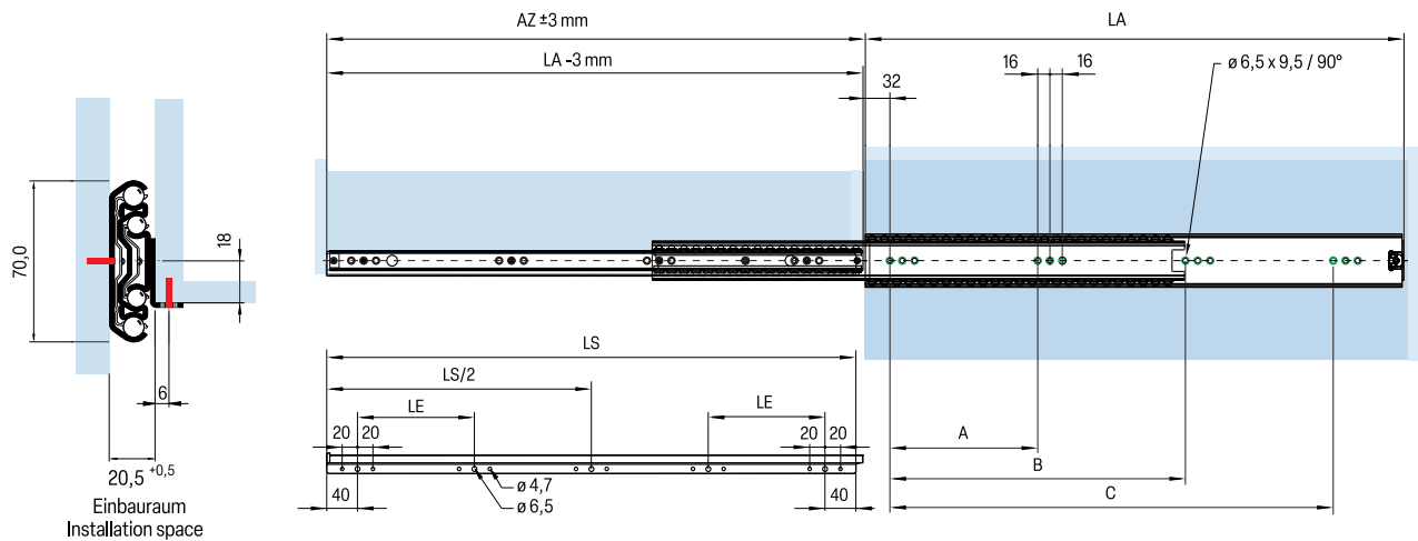
Befestigung mit M5-Senkkopfschrauben (Kopfhöhe 2,5 mm) oder Euro-Schrauben (Senkkopf Höhe 1,5 mm) Fixing with M5 countersunk screws (screw head height 2,5 mm) or Euro screws (countersunk head height 1,5 mm)
